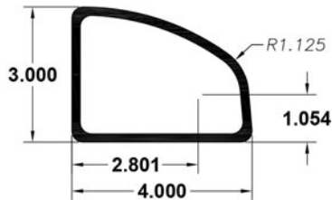
D-Tube/Frame x 24' 6063-T52 52-63-14618W (NC) 4.000 x 3.000
